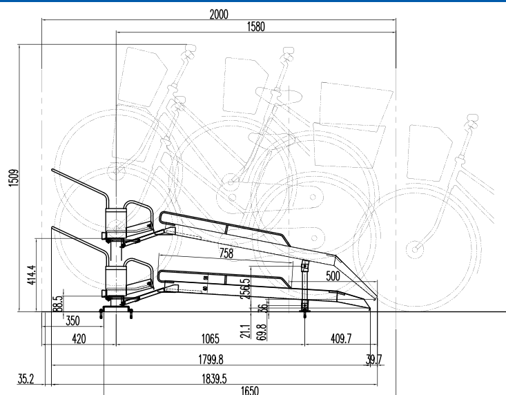
側面図
